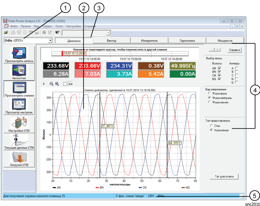
Рисунок 5. Экран текущих данных
