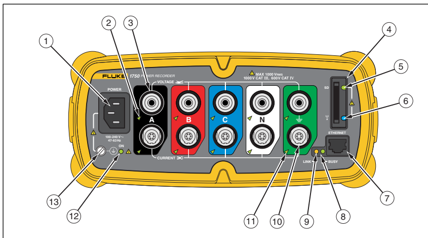
Рисунок 1. Fluke 1750 Power Recorder
