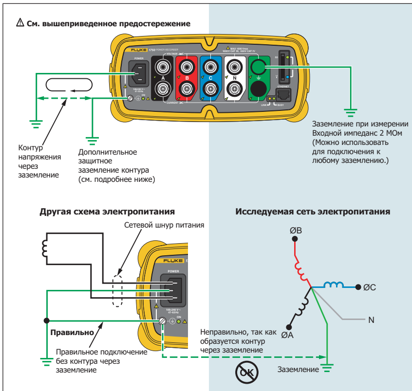
Рис. 2. Подключение дополнительной клеммы заземления
