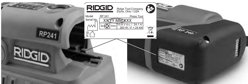
Figur 3 – Verktøyet serienummer - Tallene i sirkelene angir år og måned for produksjon. (YY = år, MM = måned).
