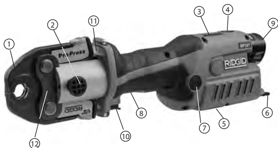
Figur 2 – RIDGID RP 241 Pressverktyg och Compact Series-käft
