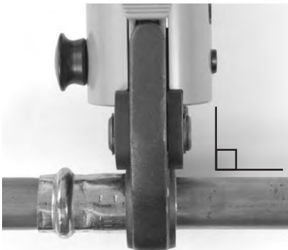
Obrázek 8 – Čelisti kolmo na armaturu
