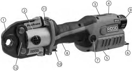
Figur 2 – Presseværktøj RP 241 fra RIDGID og Compact series kæbe
