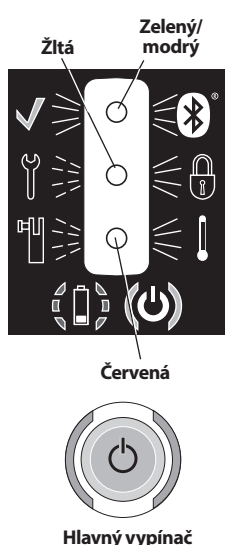
Obrázok 4 – Tabuľka ovládacích prvkov
