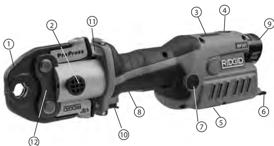
Figura 2 – Pressatrice RP 241 e Ganascia della Serie Compact RIDGID
