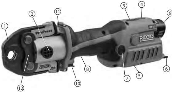
Figura 2 – Mașina unealtă de presare RIDGID RP 241 și falca Compact Series
