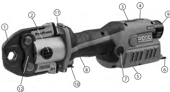
Rysunek 2 – Zagniatarca RIDGID RP 241 i szczęka serii Compact
