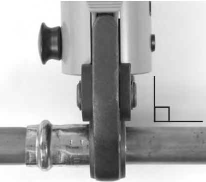
8. ábra – A pofák merőlegesen állnak a szerelvényre
