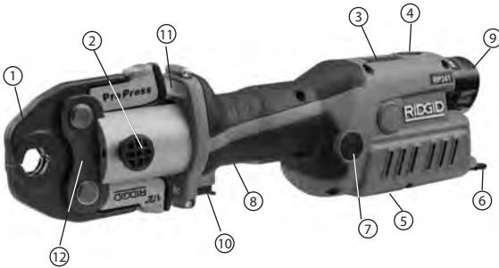
2. ábra – RIDGID RP 241 présszerszám kompakt sorozatú szorítófókkal
