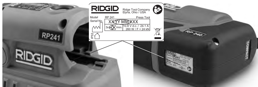
Obrázok 3 – Výrobné číslo zariadenia - Zakrúžkované číslice znamenajú rok a mesiac výroby. (RR = rok, MM = mesiac).
