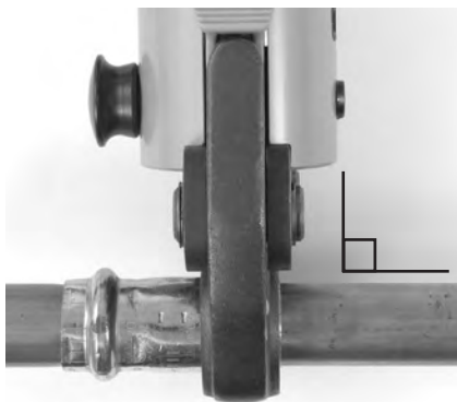
Slika 8 – Čeljusti pravokotno na nastavek
